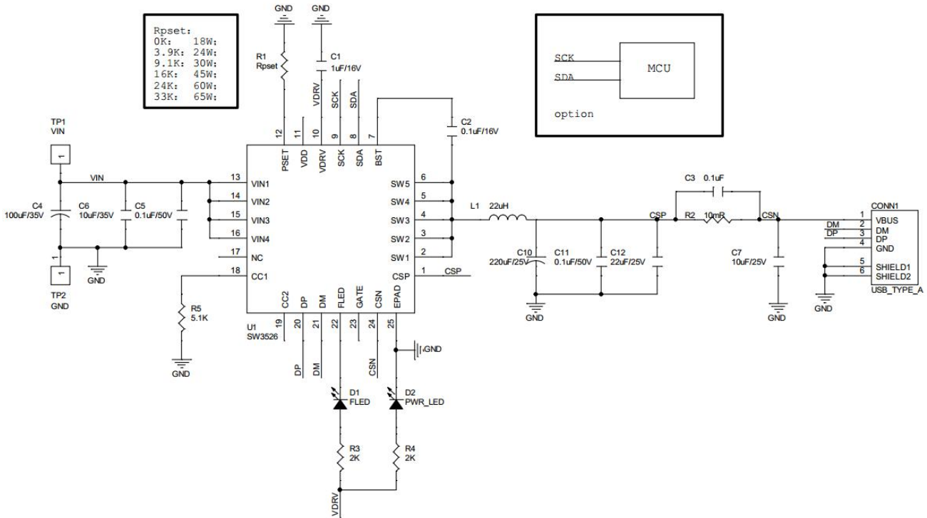
Type-A 口输出应用
