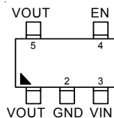
SOT-23-5
